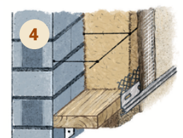
ITE BLOCPAILLE / ENDUIT TERRE-CHAUX
